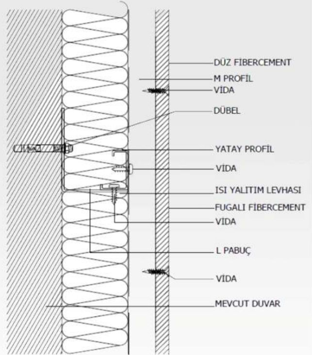
DÜZ FİBERCEMENT UYGULAMA
